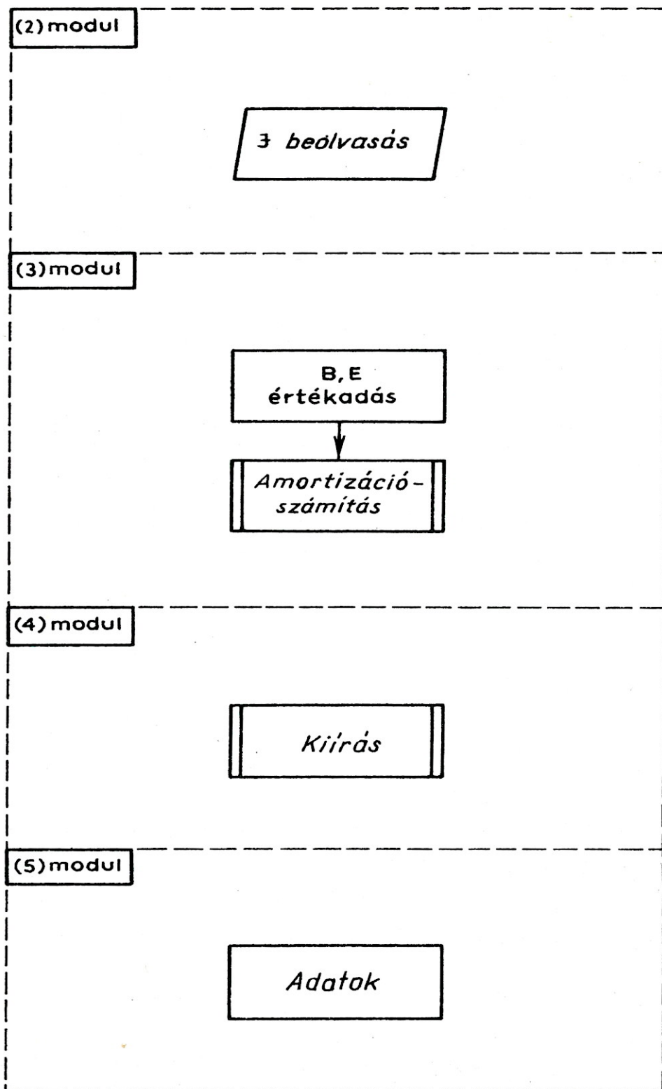
38. ábra. A 2.1 feladat szubrutinjai
