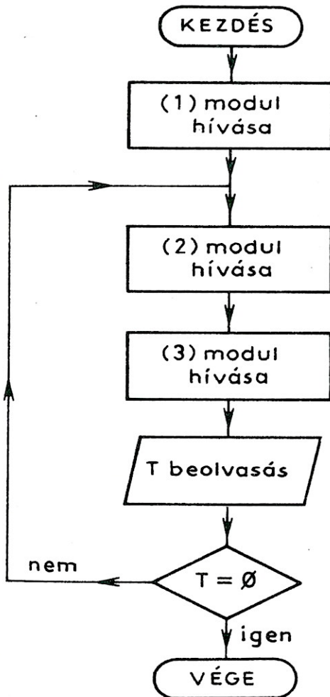
37. ábra. A (1) modul folyamata
