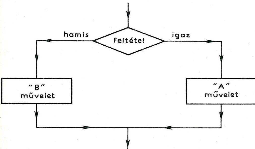
13. ábra. Az IF THEN ELSE típusú szerkezet
