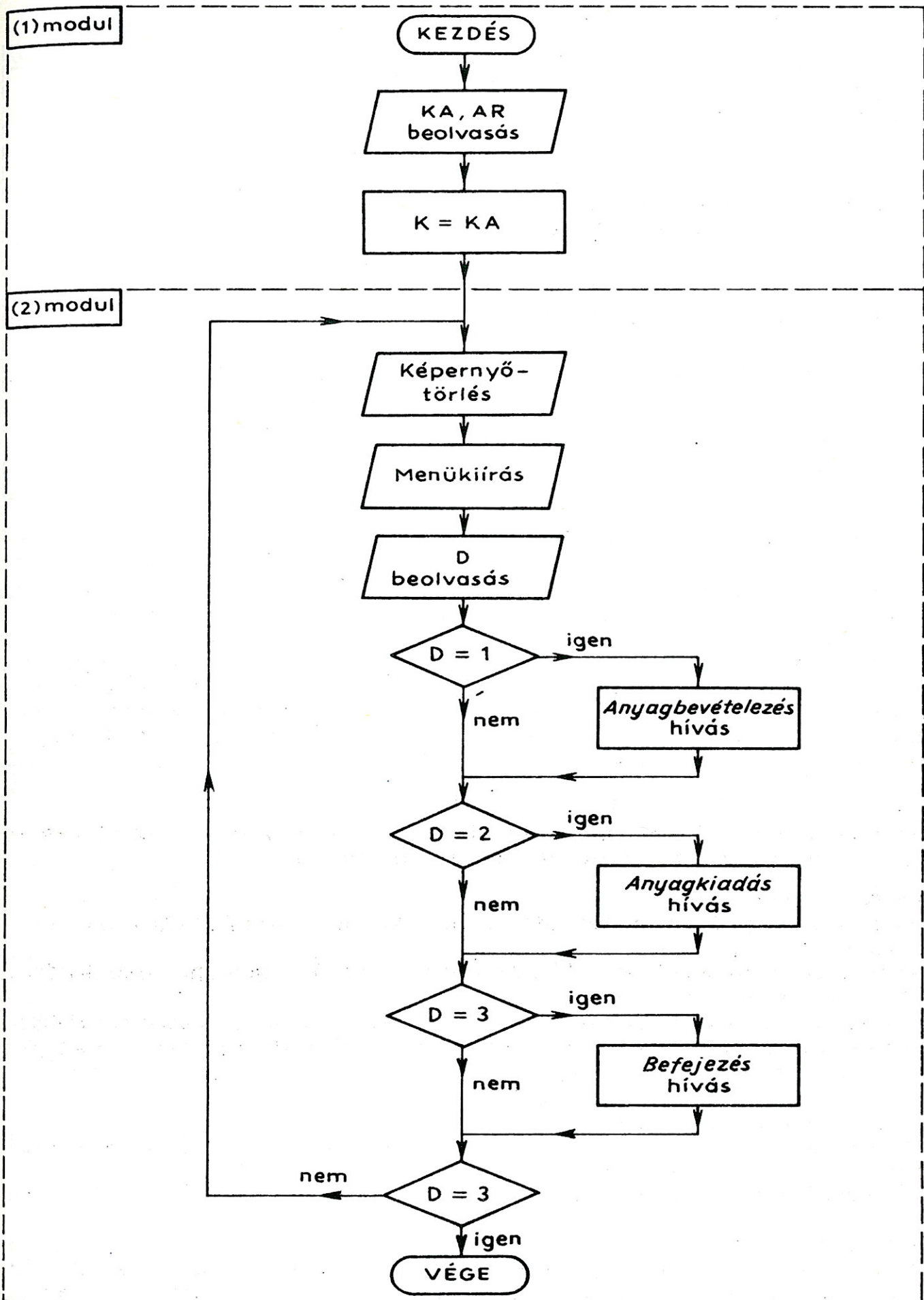
46. ábra. A (1) és (2) modul folyamata
