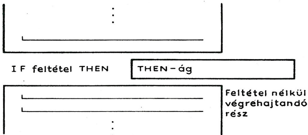
23. ábra. Az egyszerűsített IF THEN szerkezet
