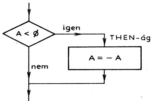
56. ábra. Abszolút érték meghatározása
