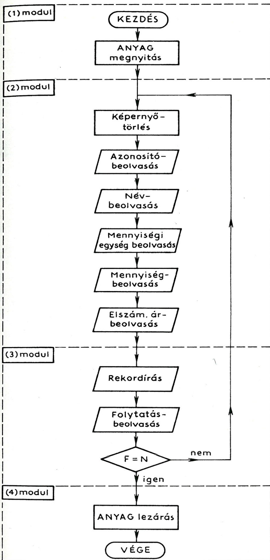
94. ábra. A program folyamata
