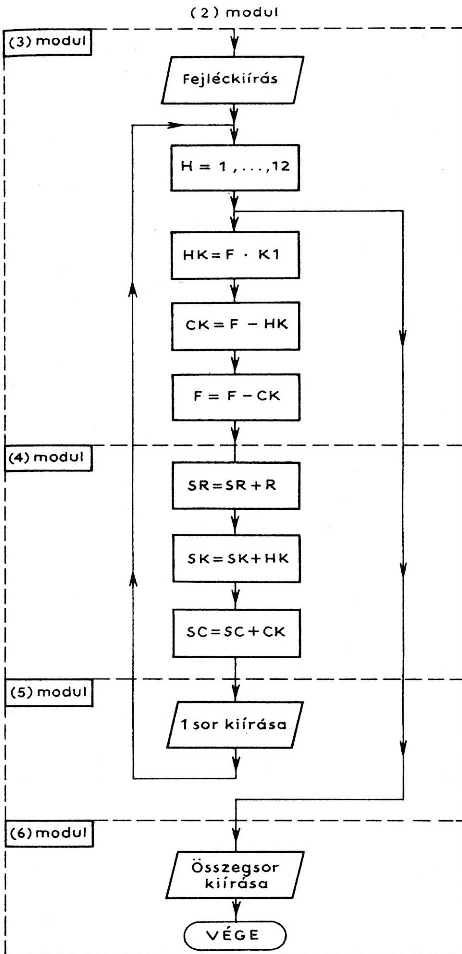
60. ábra. A (3), (4), (5) és (6) modulok folyamata
