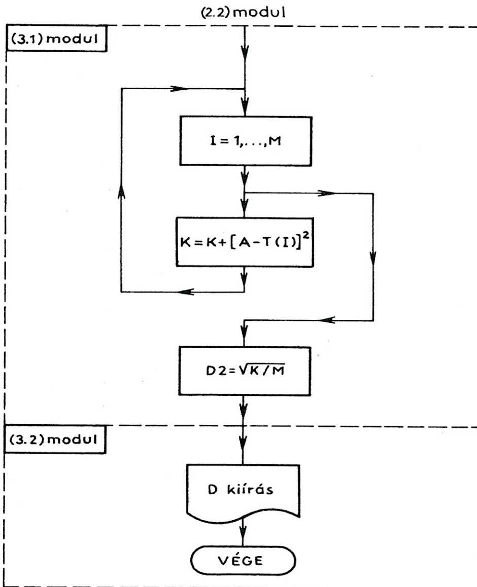
65. ábra. A (3.1) és (3.2) modul folyamata
