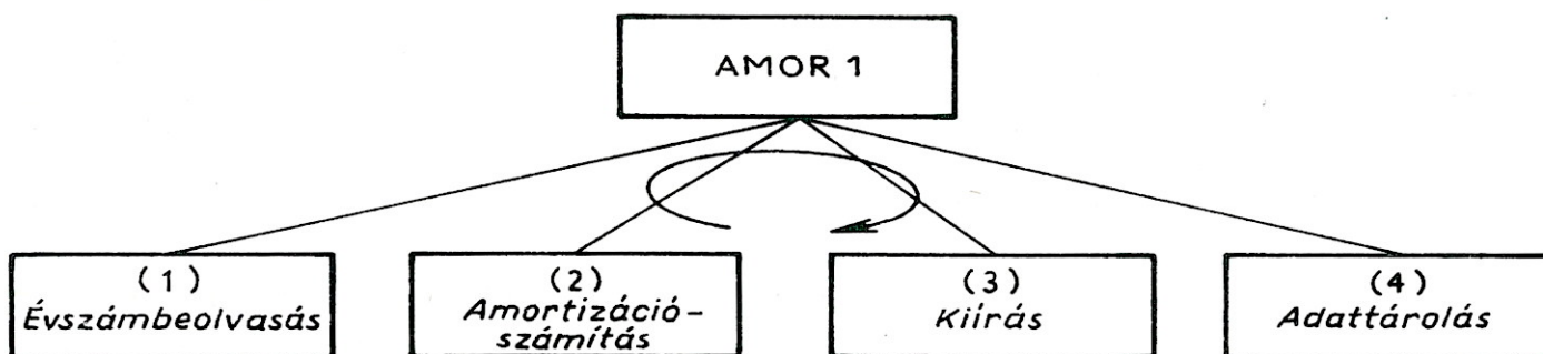
36. ábra. A módosított 2. feladat programjának szerkezete
