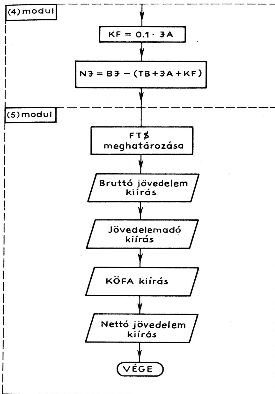
43. ábra. A (4) és (5) modulok folyamatai
