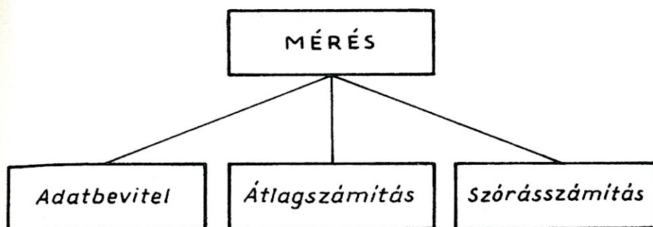
61. ábra. A 9. feladat programjának modulszerkezete
