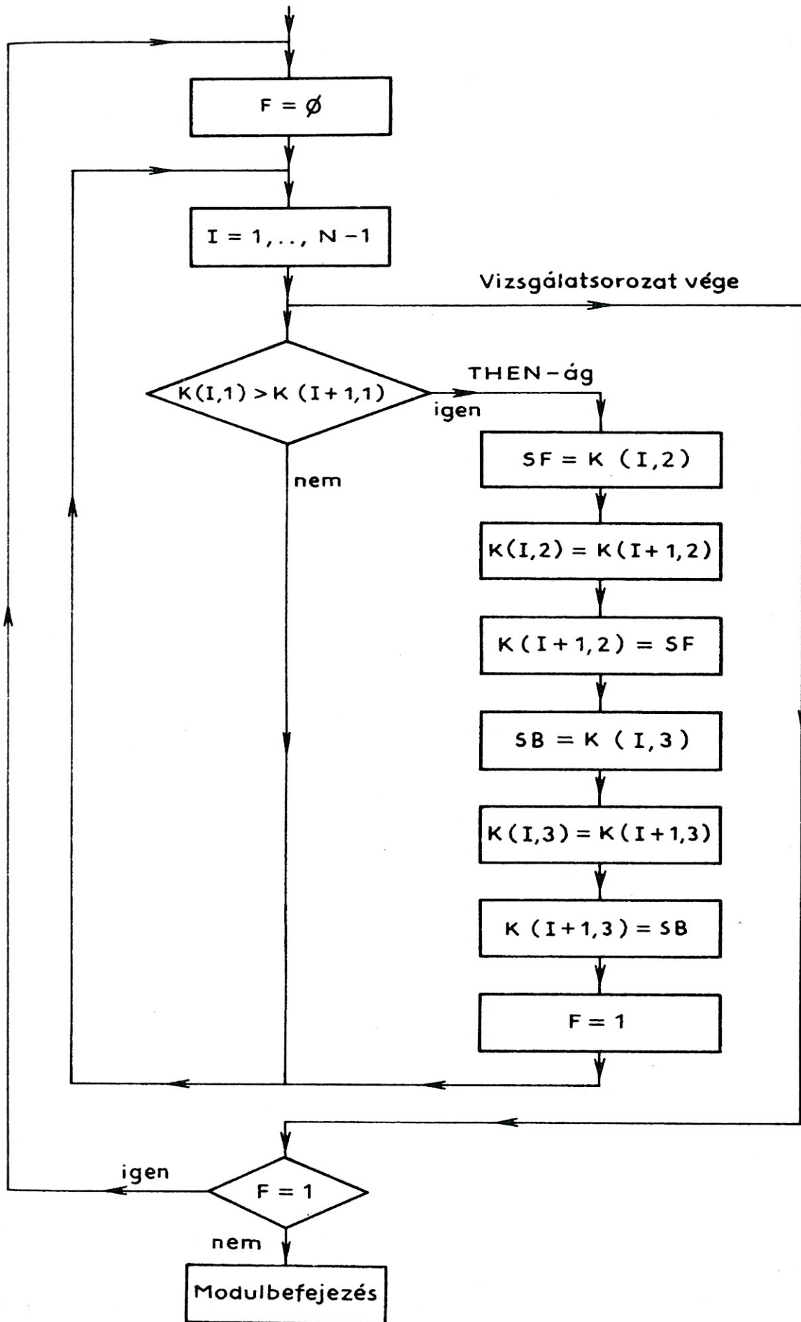
74. ábra. A (6) modul folyamata
