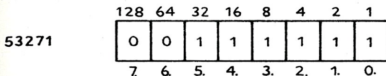
119. ábra. A kétszerező bájt tartalma
