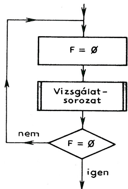
73. ábra. A vizsgálat-sorozatot tartalmazó ciklus
