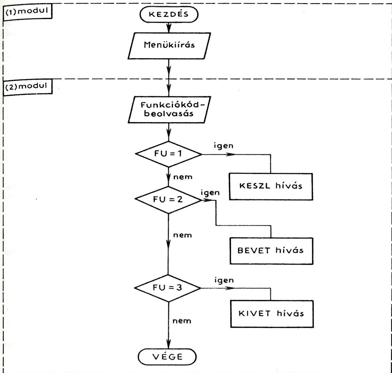
99. ábra. A MENU program folyamata
