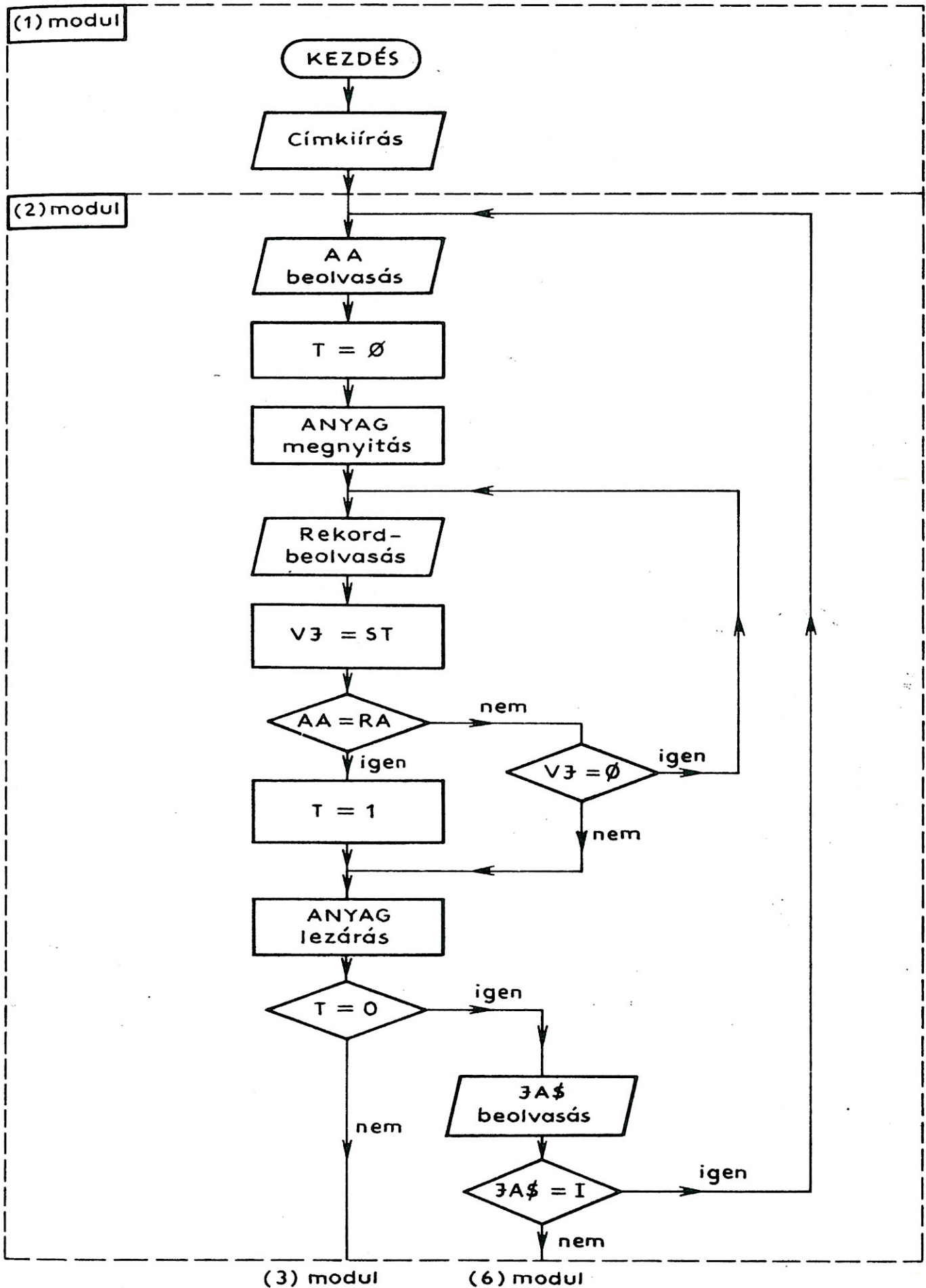
100. ábra. Az (1) és (2) modul folyamata
