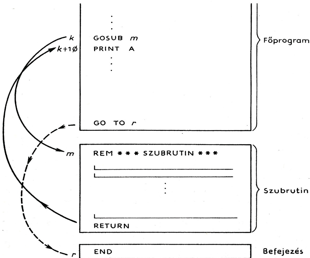
35. ábra. A szubrutint tartalmazó program
