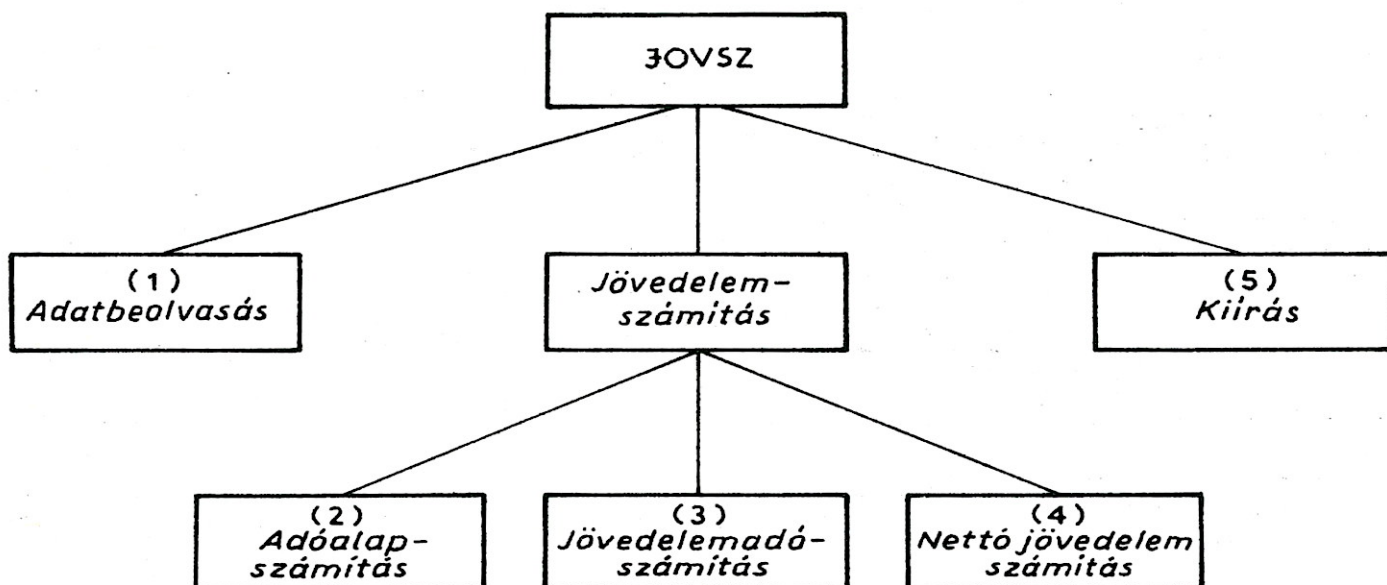
40. ábra. A 3. feladat modul szerkezete
