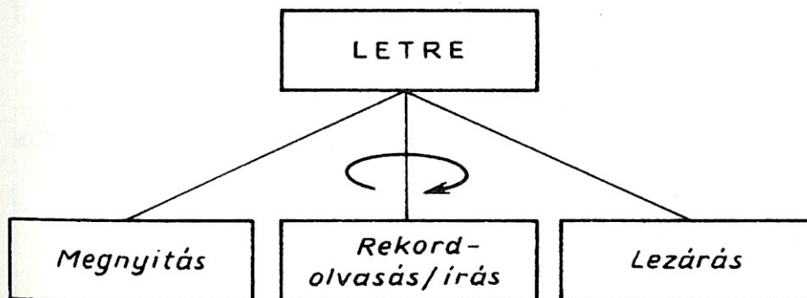
92. ábra. A létrehozó program szerkezete
