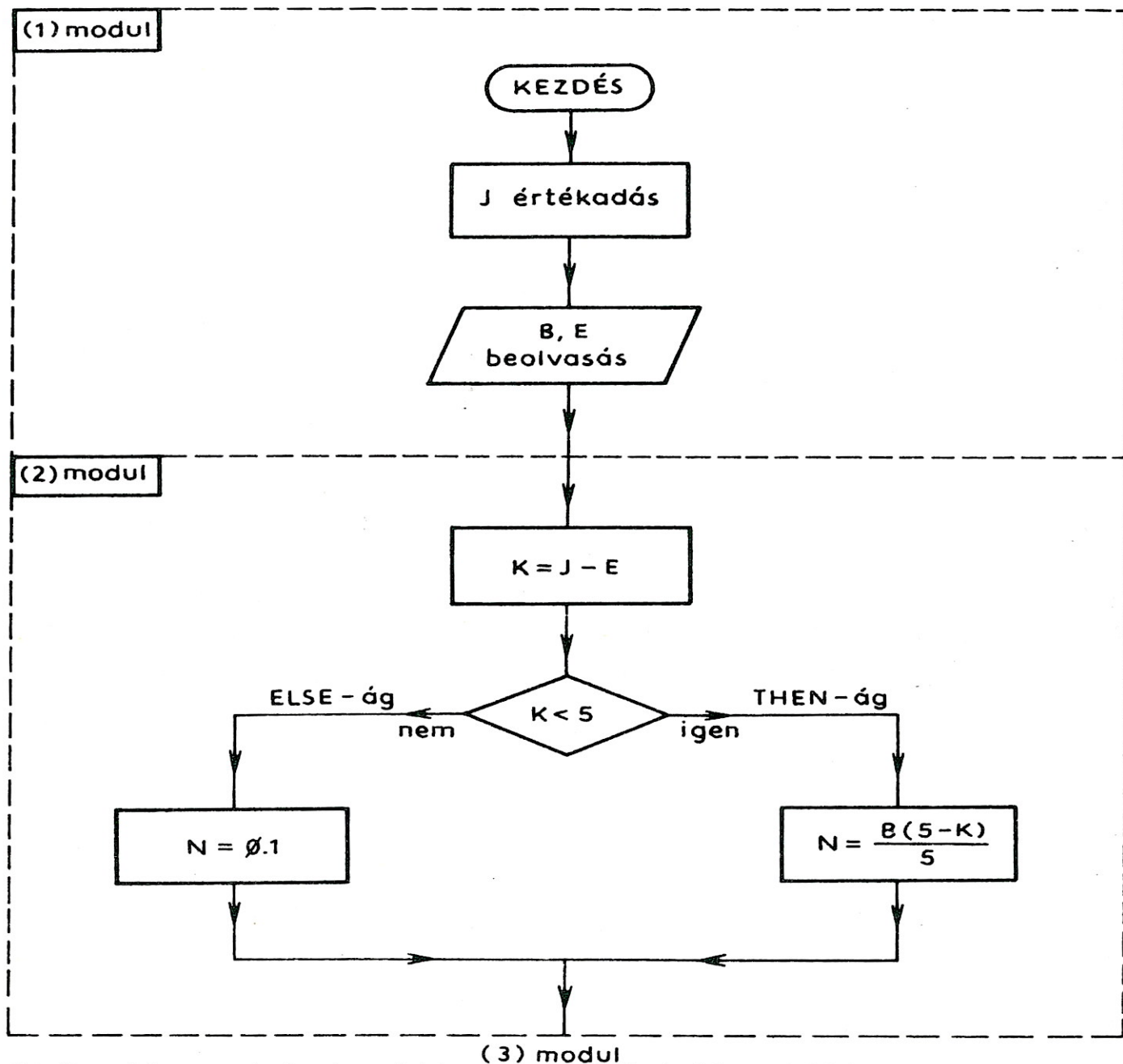
31. ábra. A bemeneti adatok modul és az amortizációs számítás modul folyamata
