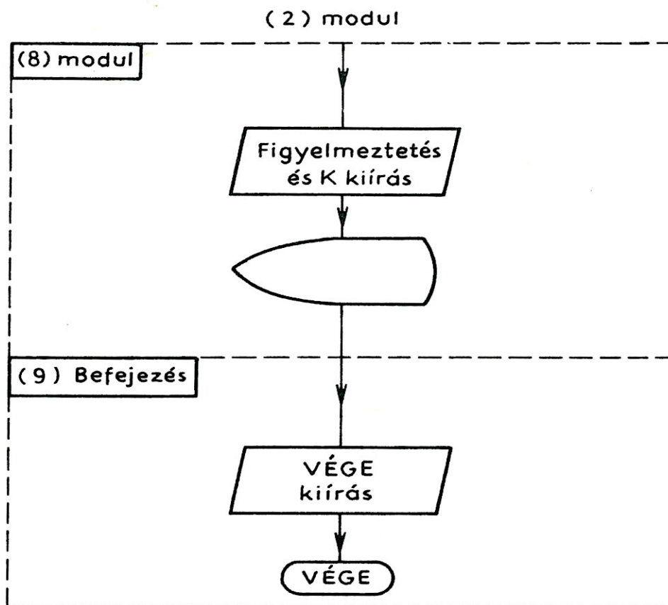
49. ábra. A befejező modulok folyamata
