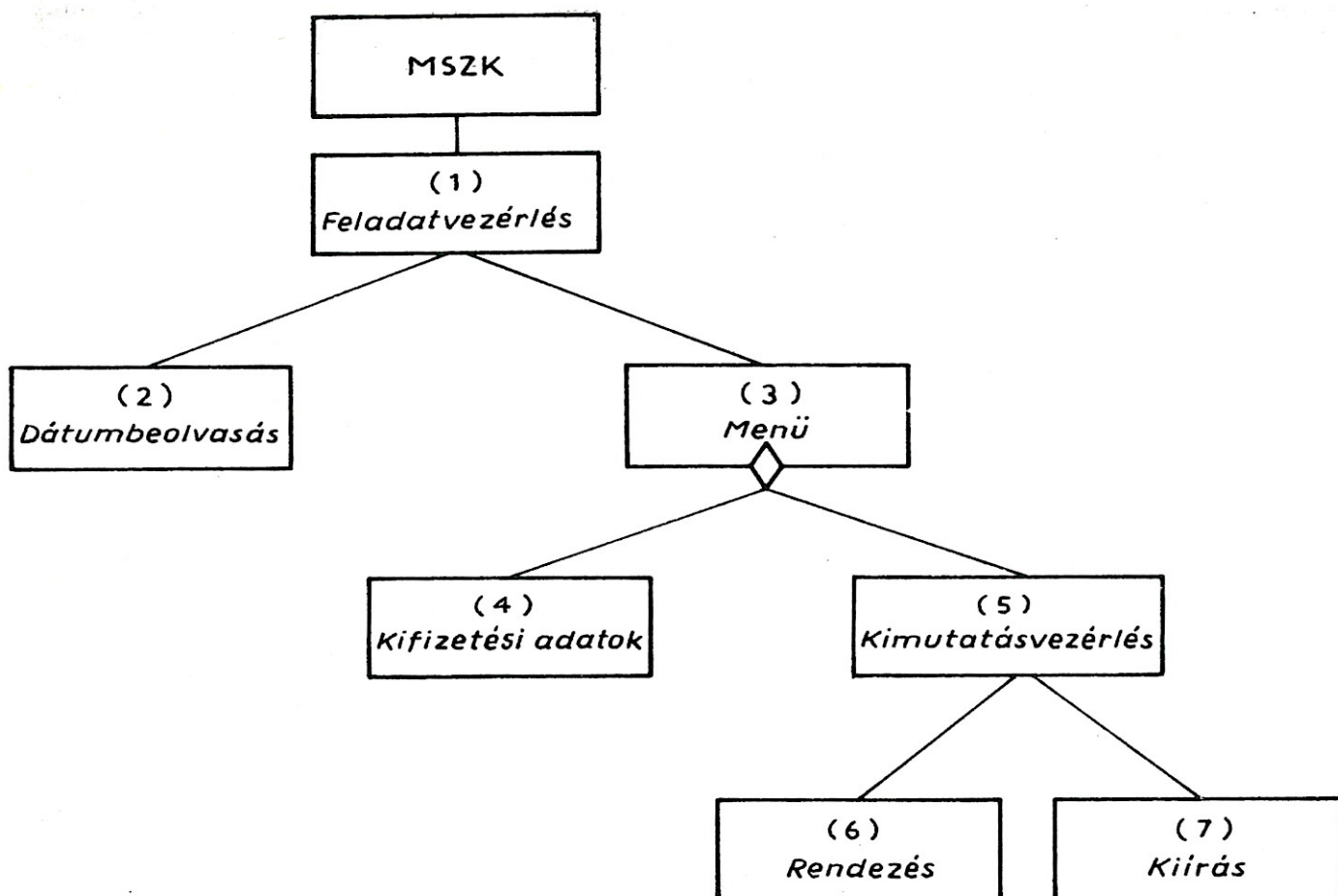
67. ábra. A 7. feladat modulszerkezete
