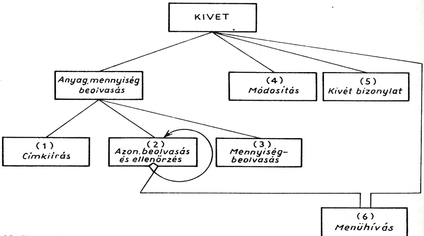
98. ábra. A KIVET program terve
