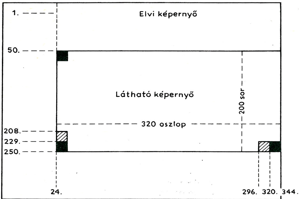
106. ábra. Foltok elhelyezése a képernyőn
