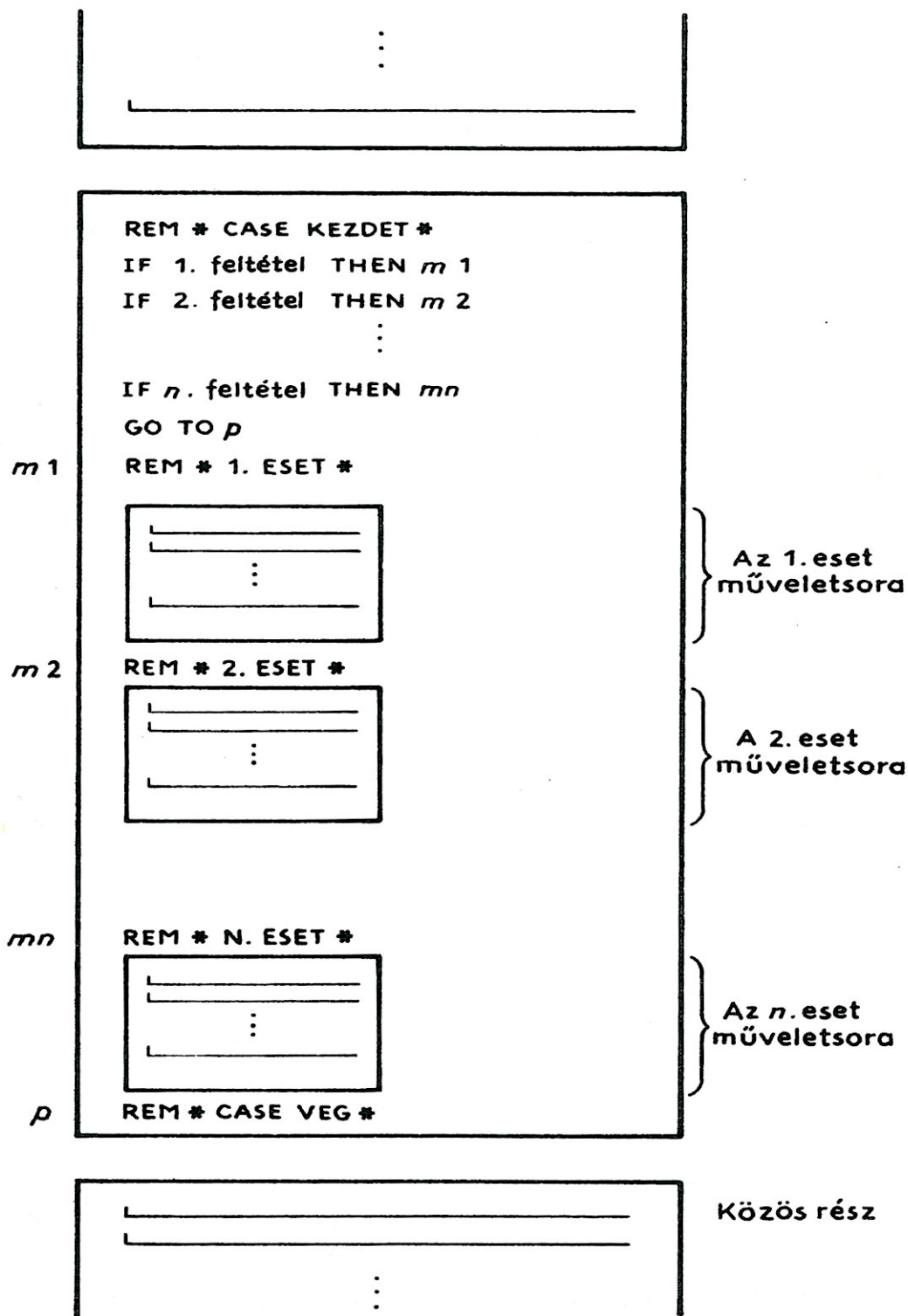
28. ábra. A CASE szerkezet kódolása
