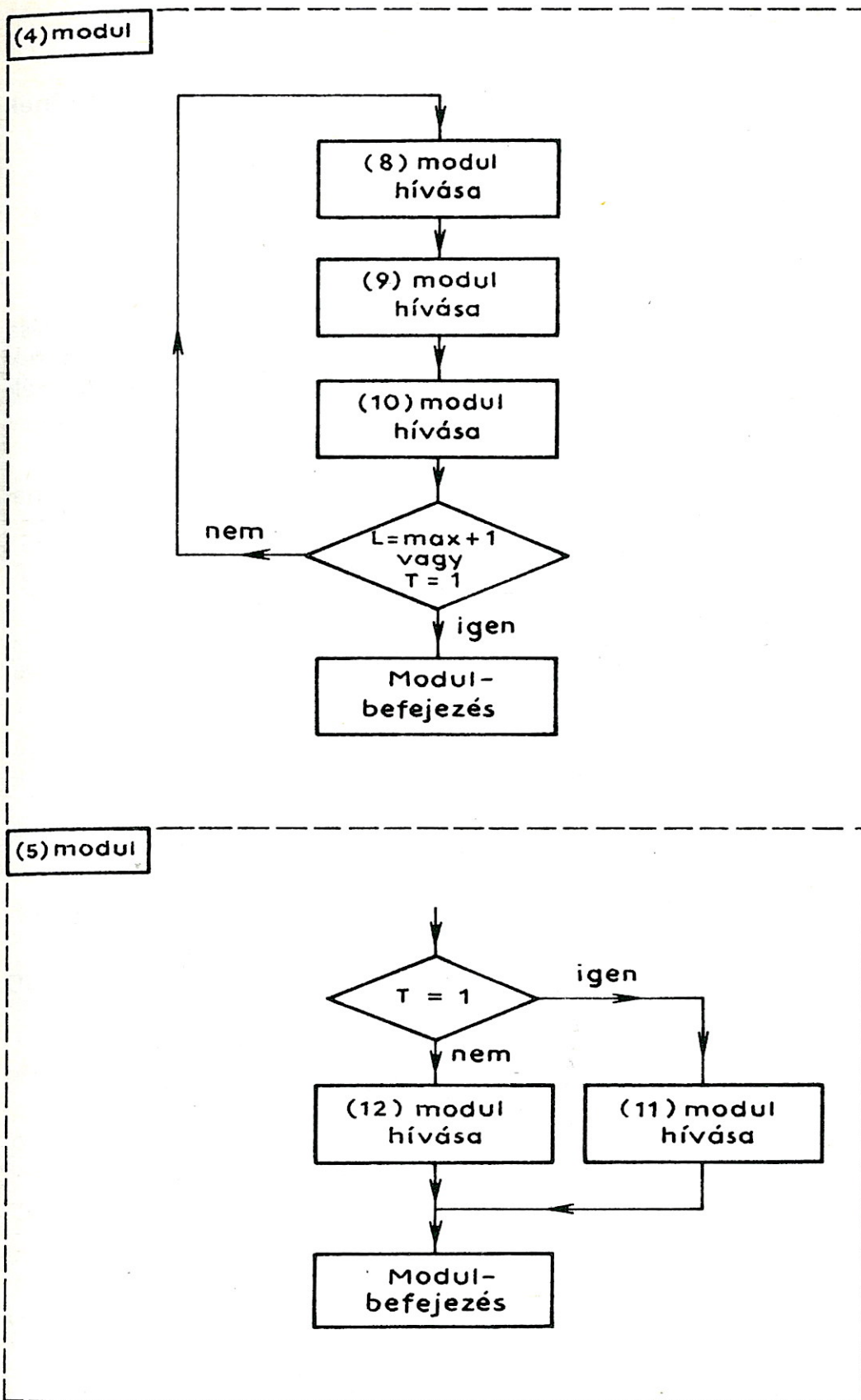
82. ábra. A (4) és (5) modulok folyamata
