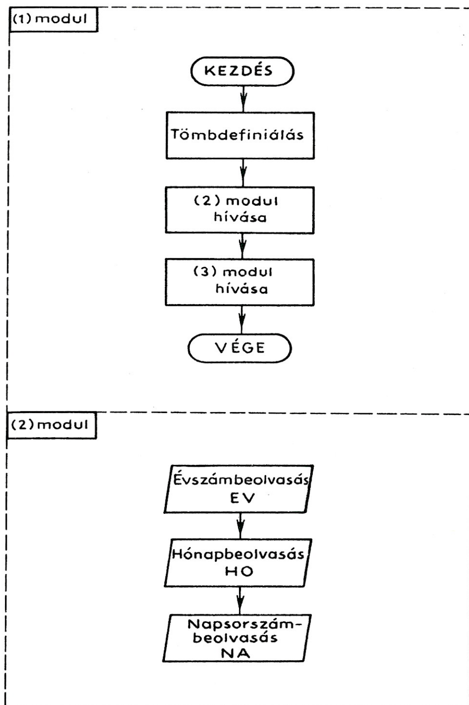
68. ábra. Az (1) és (2) modulok folyamata
