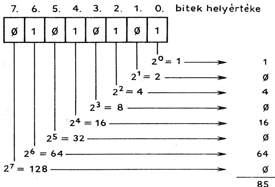
103. ábra. A bitek jelentése
