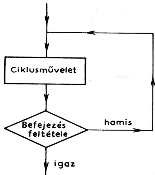
16. ábra. A hátul tesztelő ciklusszerkezet
