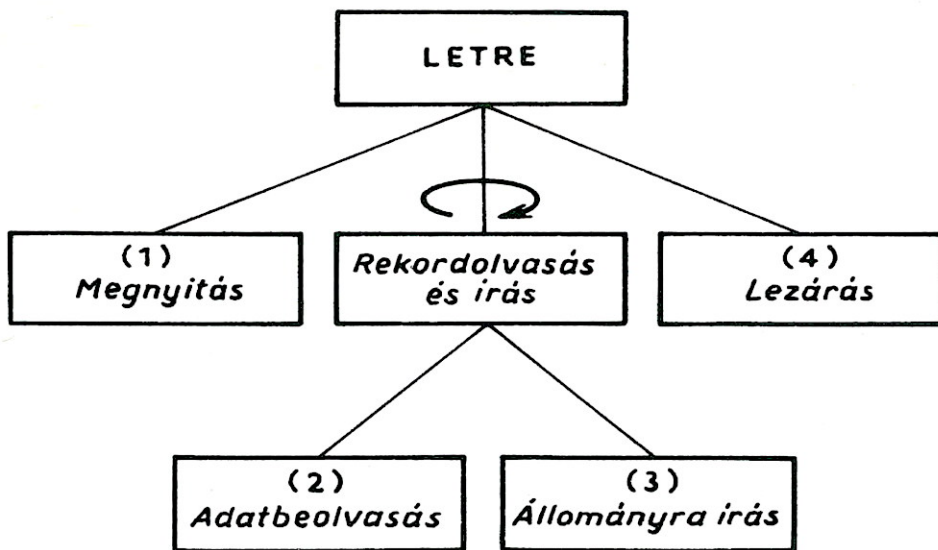
93. ábra. A program moduljai
