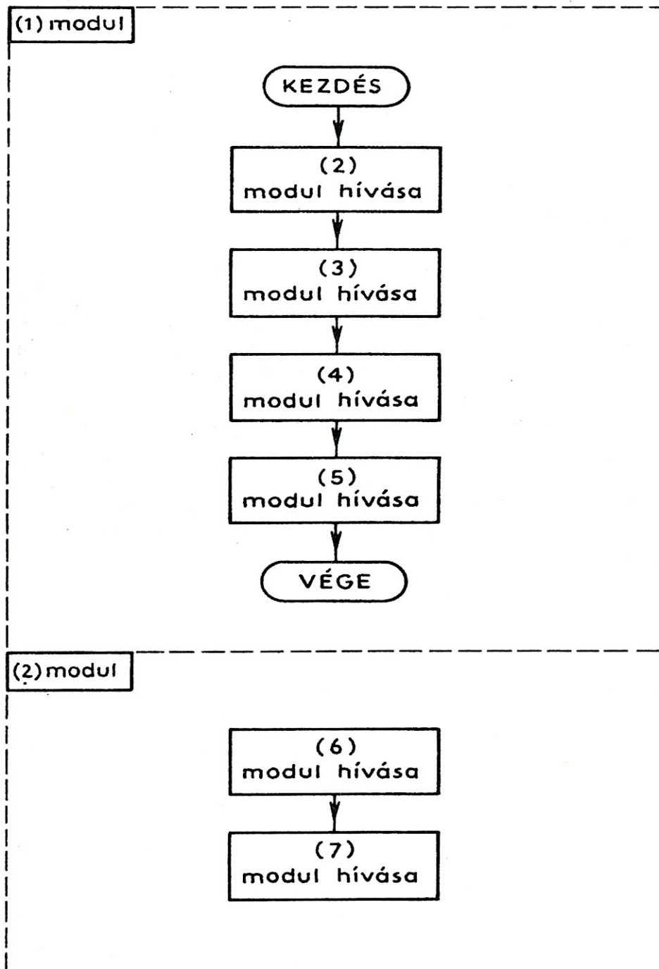
80. ábra. Az (1) és (2) modul folyamata
