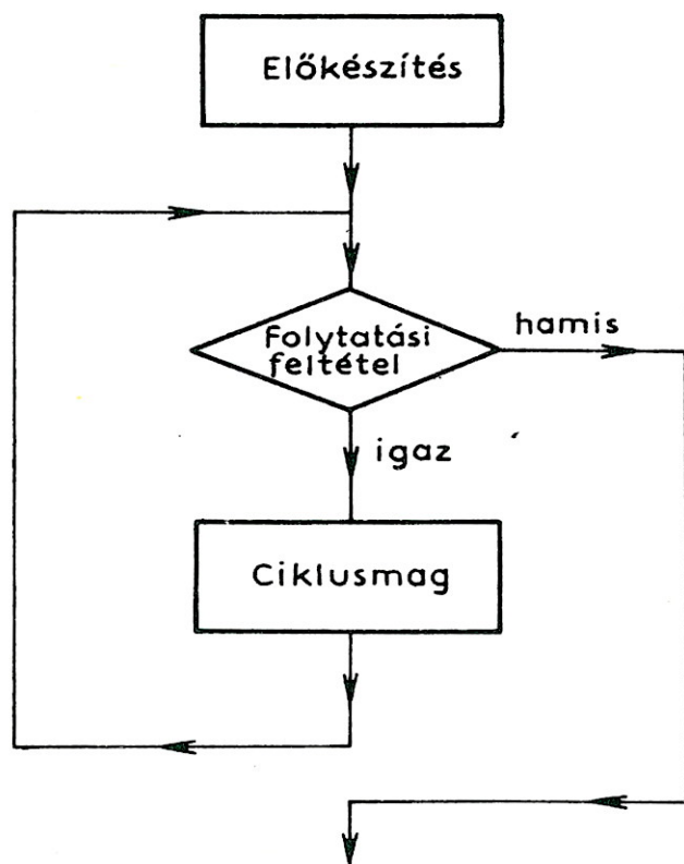
52. ábra. Az elől tesztelő típusú ciklusszerkezet
