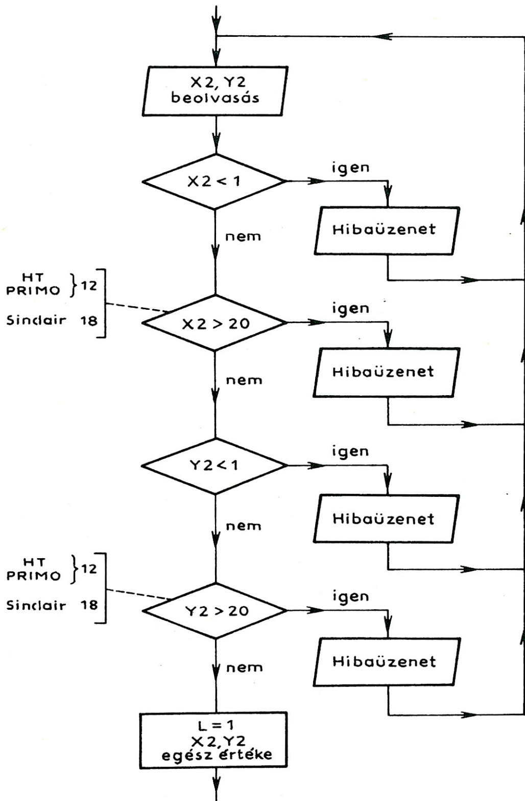
81. ábra. A (3) modul művelete
