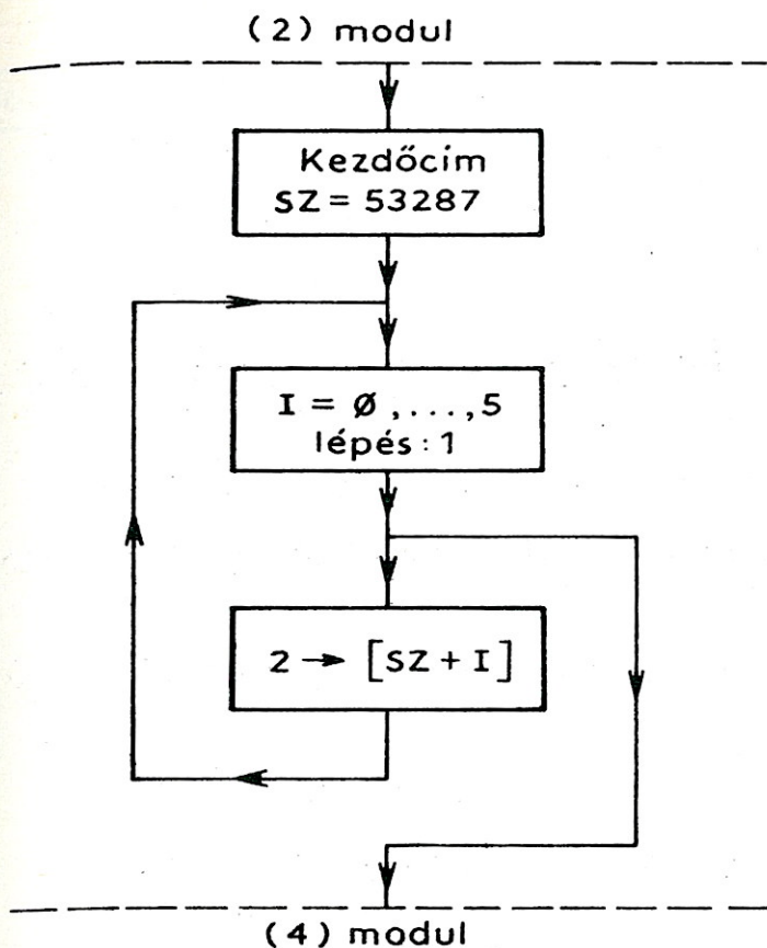
118. ábra. A (3) modul folyamata
