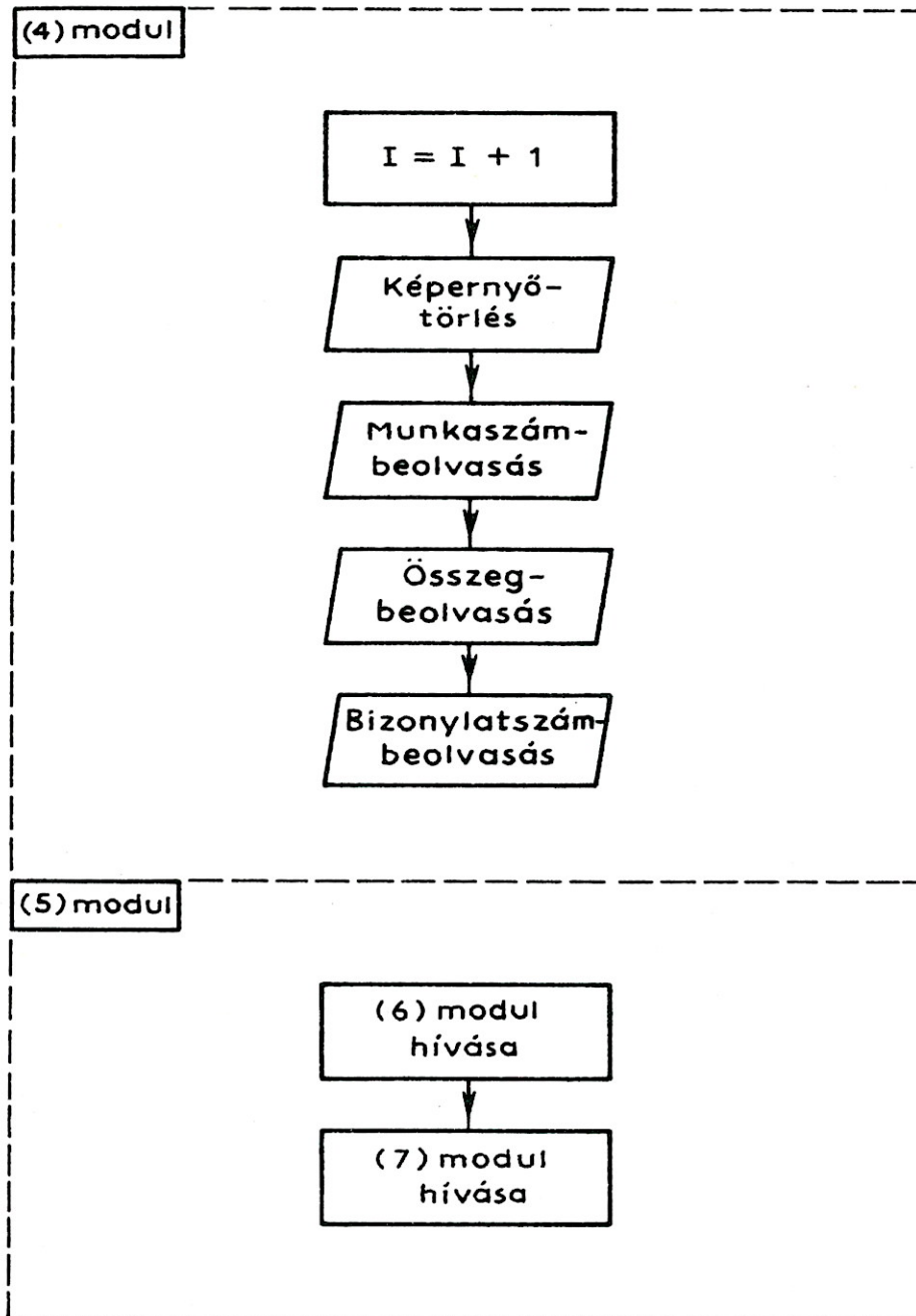
70. ábra. A (4) és (5) modul folyamata
