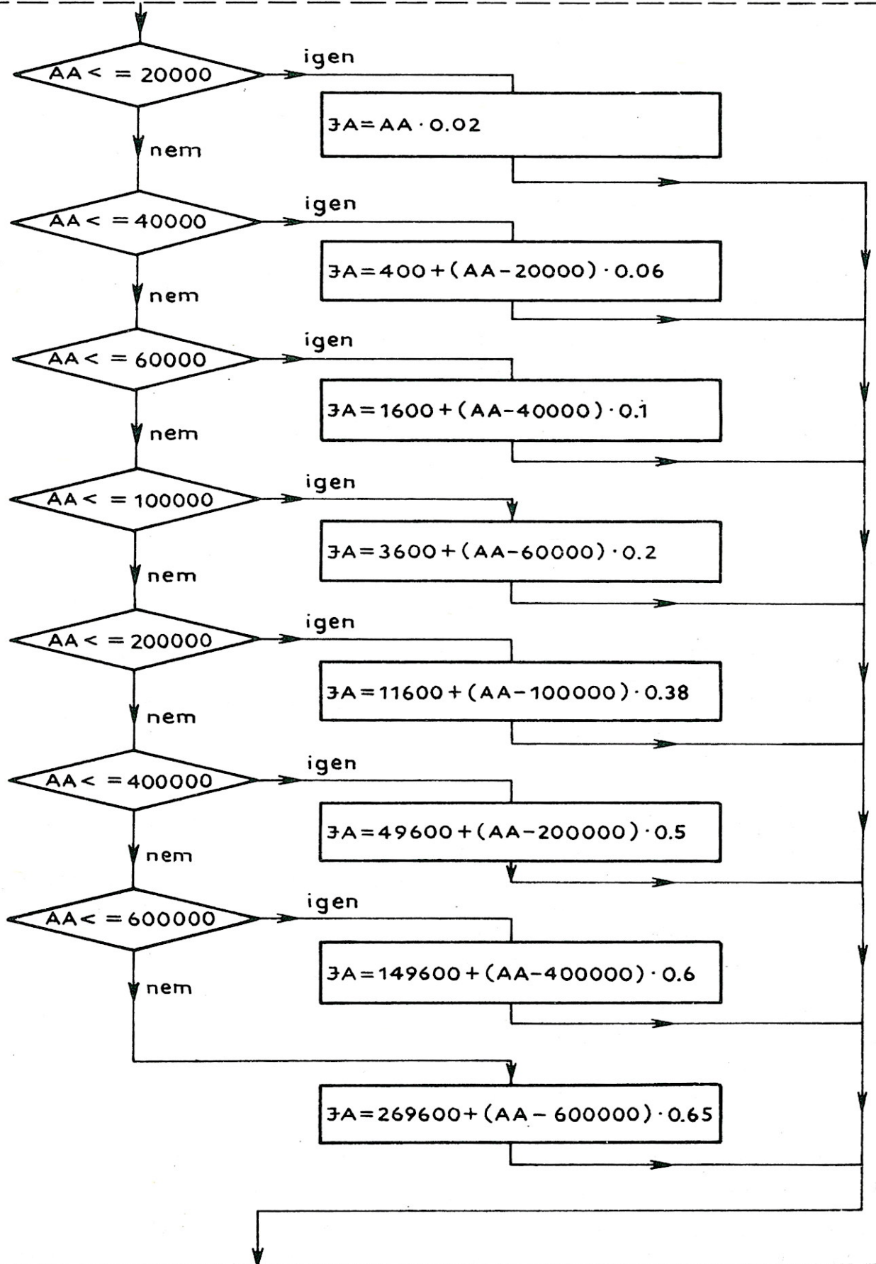
42. ábra. A (3) modul műveletei
