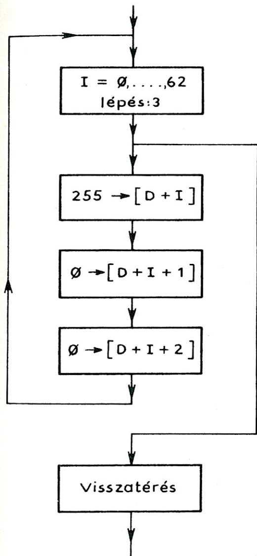
116. ábra. A teljes kitöltési szubrutin műveletei
