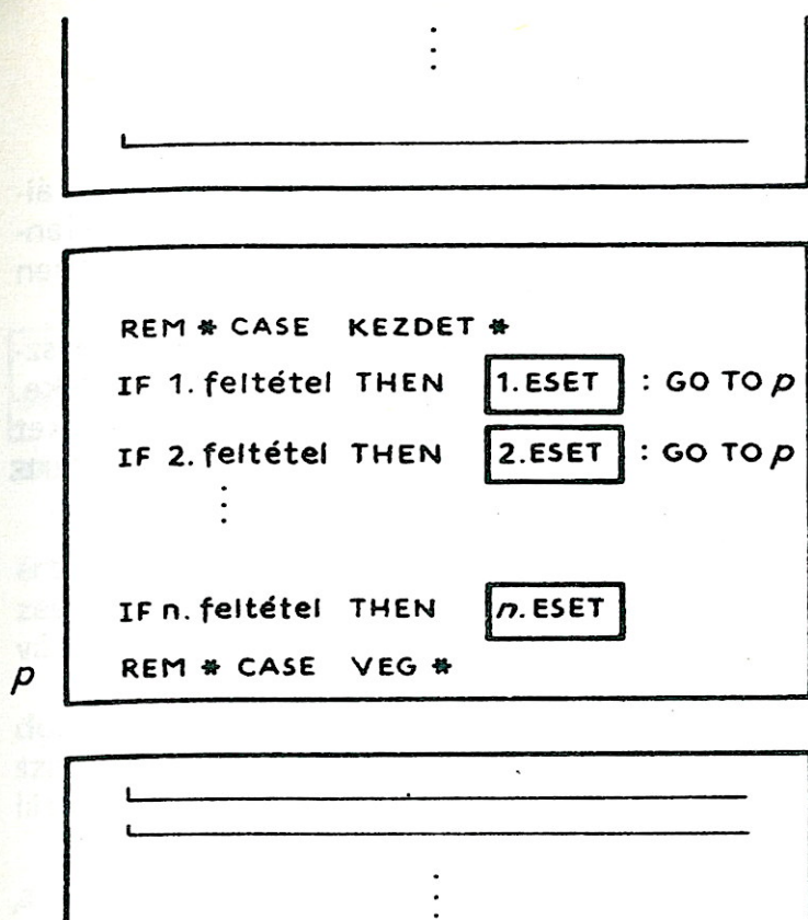
29. ábra. Az egyszerűsített CASE szerkezet
