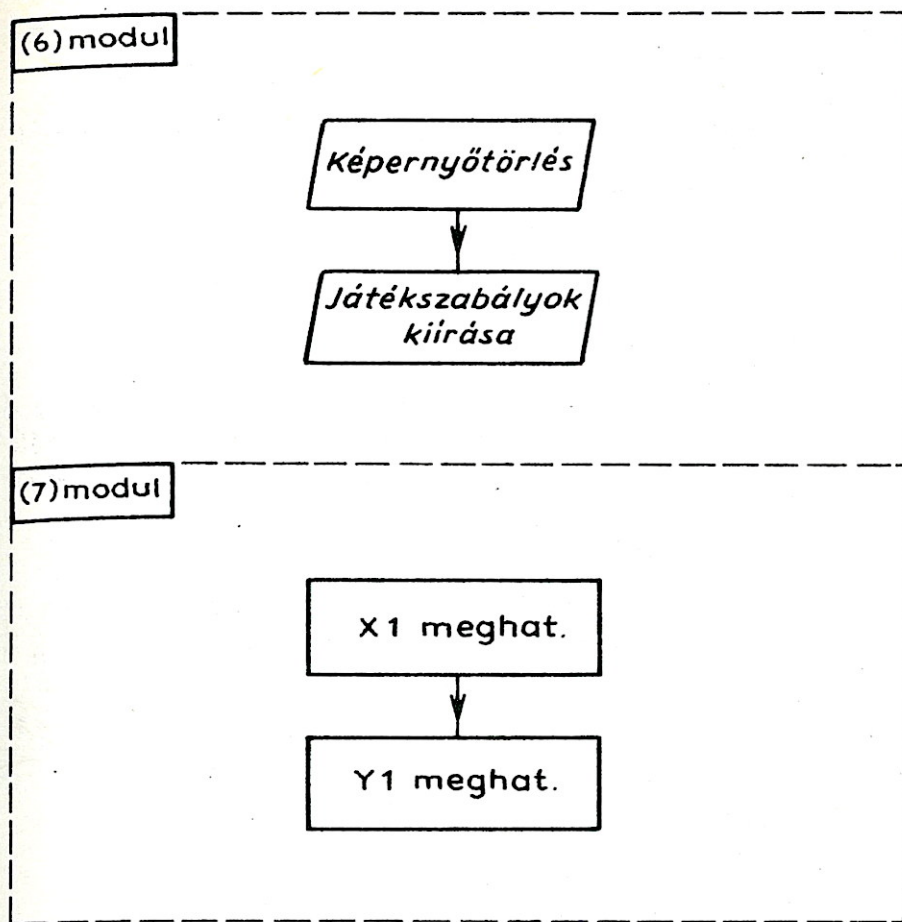
83. ábra. A (6) és a (7) modul folyamata
