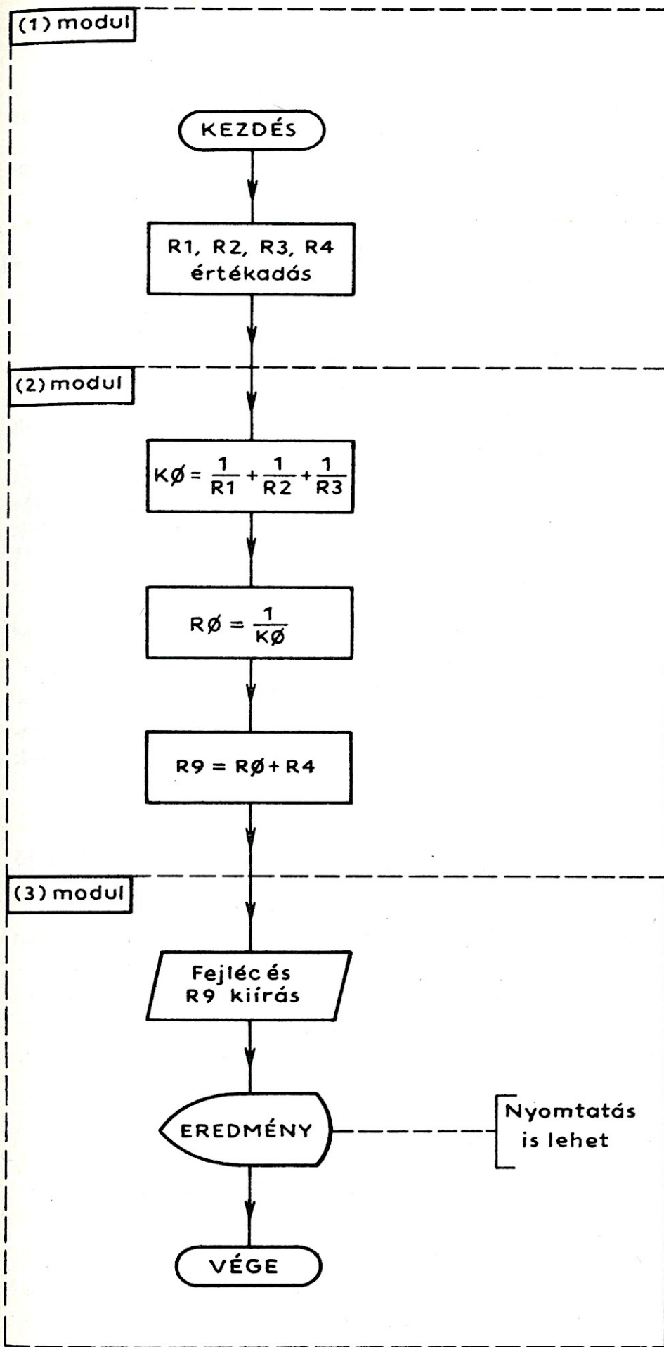
19. ábra. A modulok folyamata
