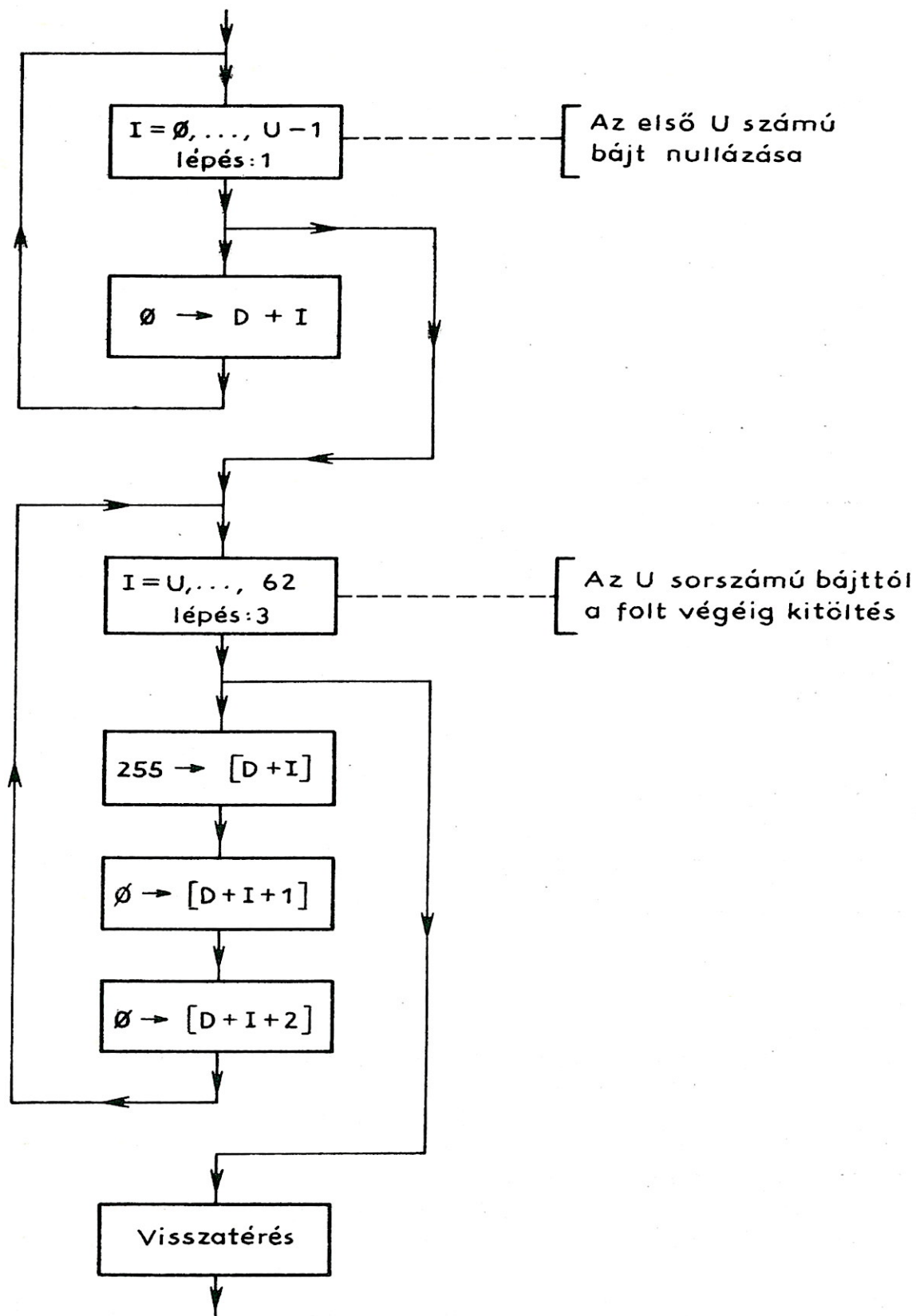
117. ábra. A részleges kitöltési szubrutin műveletei
