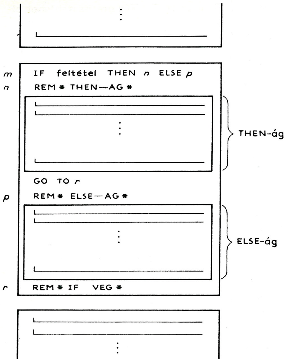
26. ábra. IF THEN ELSE szerkezet IF THEN ELSE utasítással
