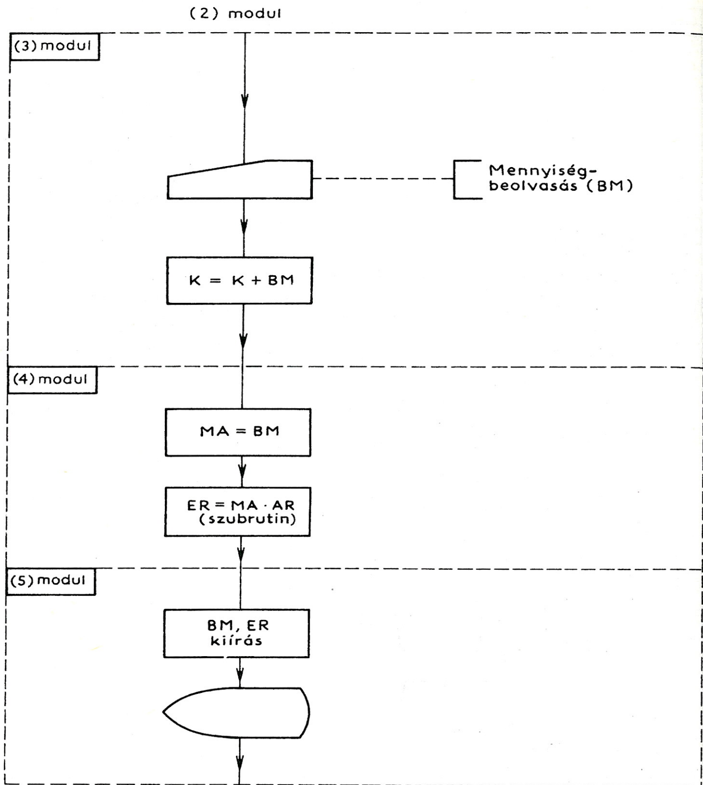
47. ábra. A bevételi modulok folyamata
