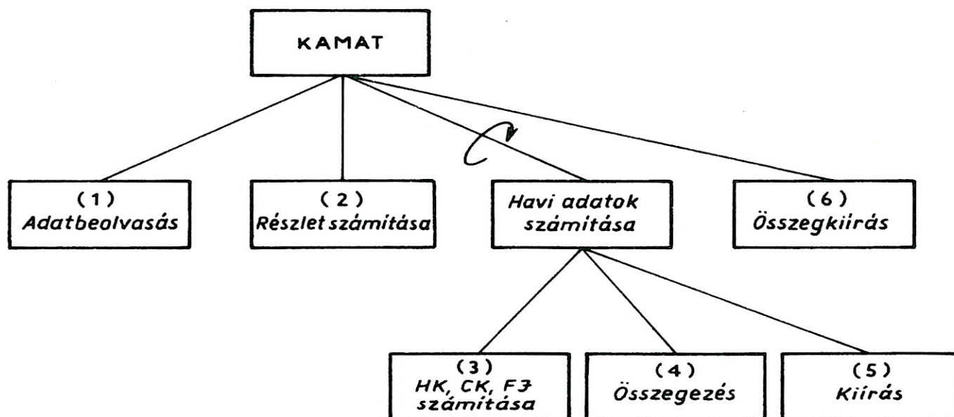
58. ábra. Az 5. feladat programjának terve
