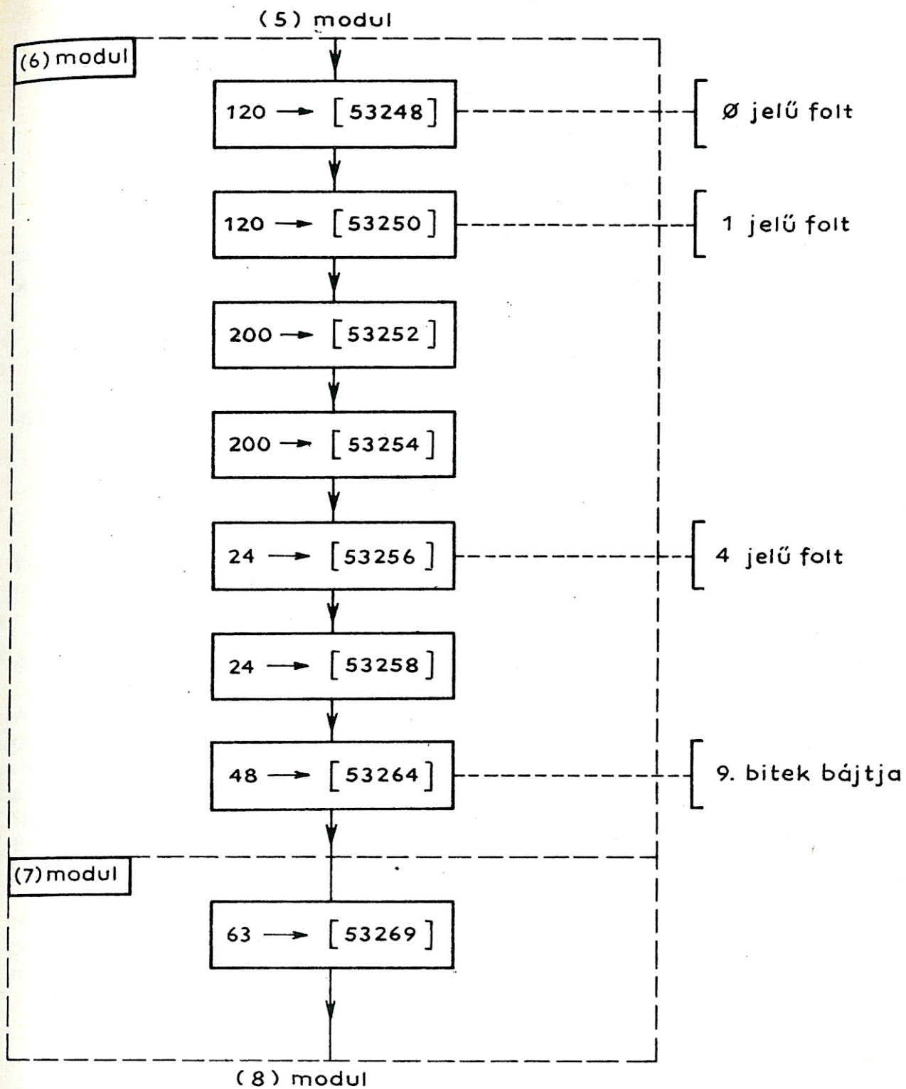
122. ábra. A (6) és (7) modul műveletei
