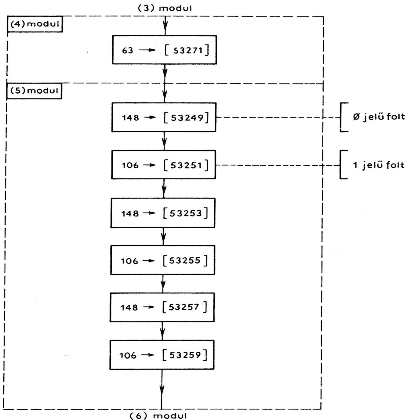
120. ábra. A (4) és (5) modul műveletei
