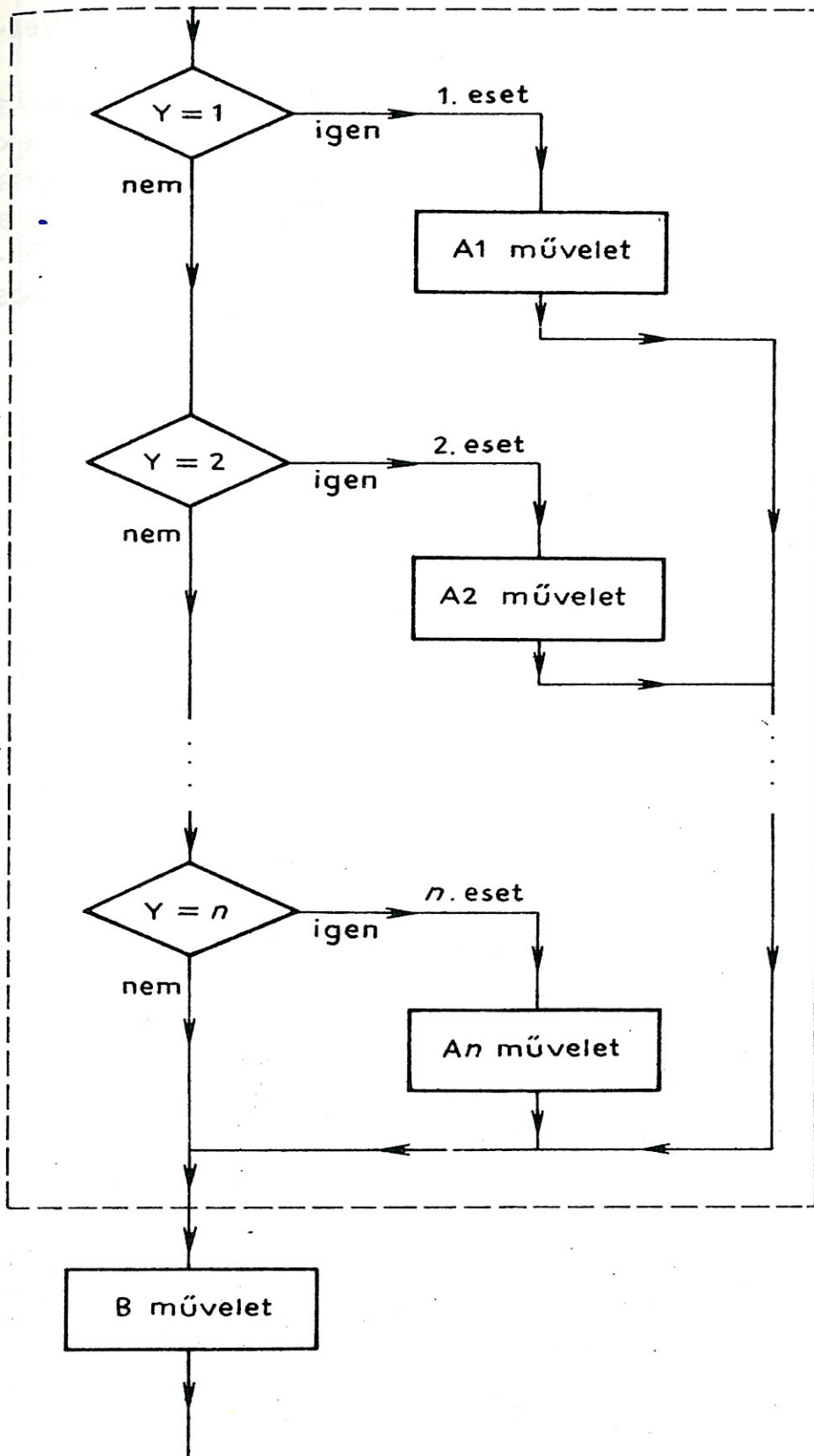
27. ábra. A CASE szerkezet
