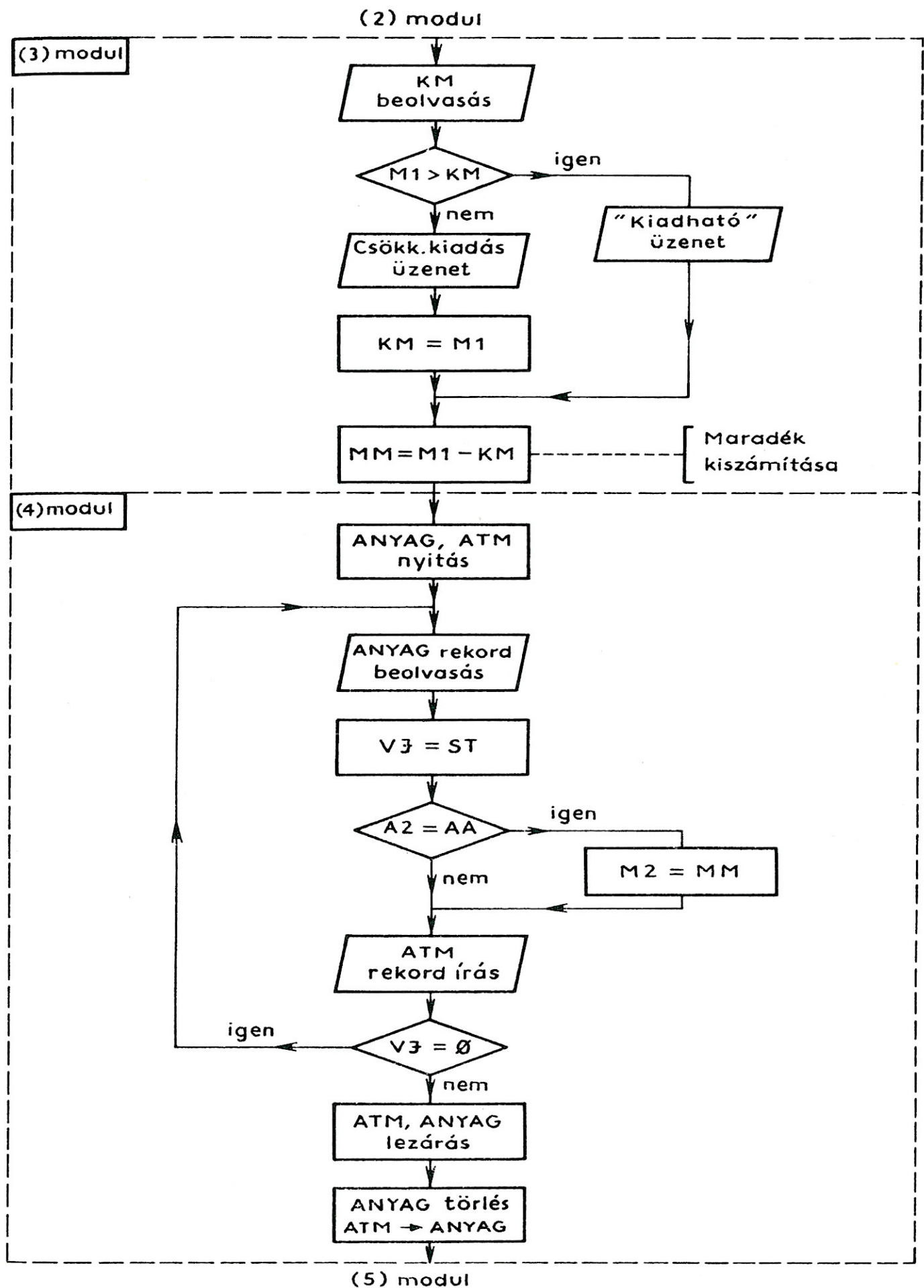
101. ábra. A (3) és (4) modulok műveletei
