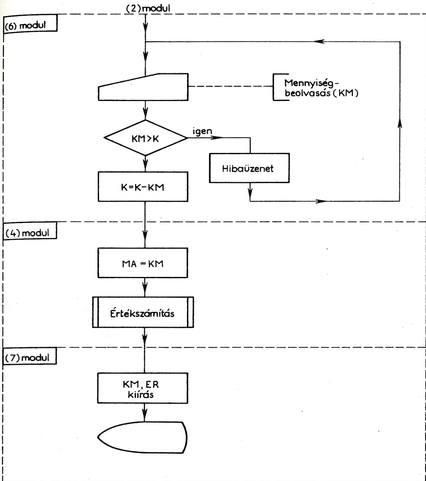
48. ábra. A kiadási modulok folyamata
