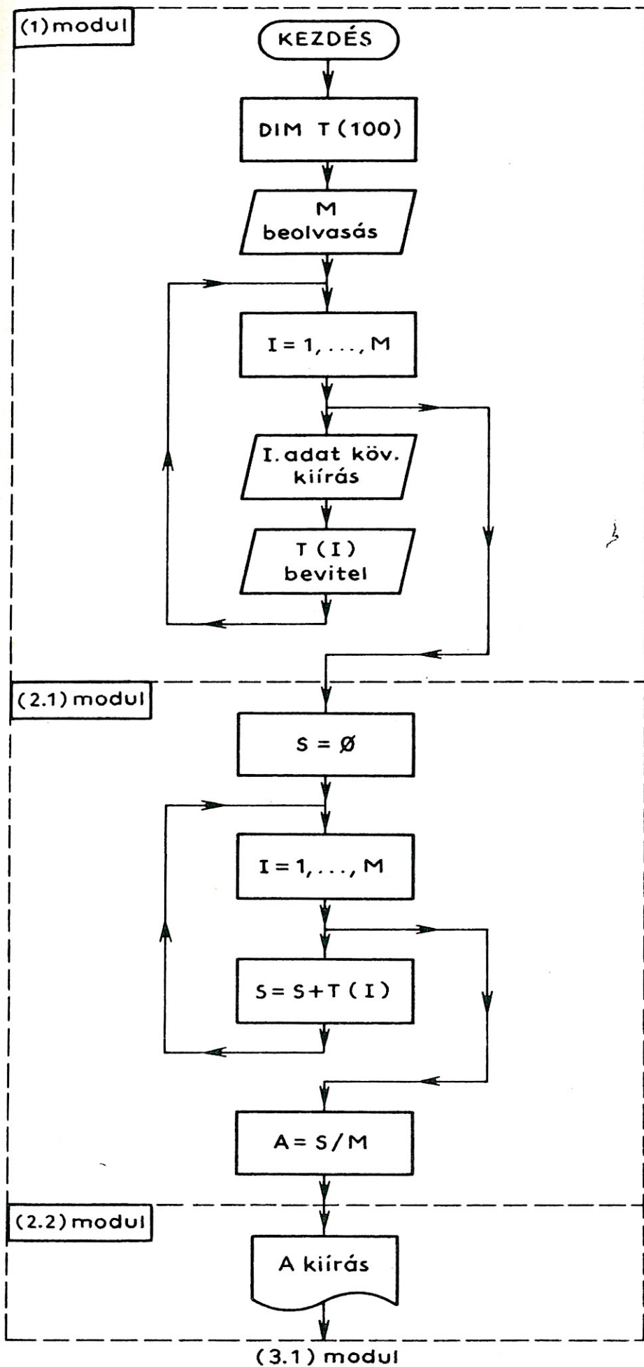
64. ábra. Az (1), (2.1) és (2.2) modul folyamata
