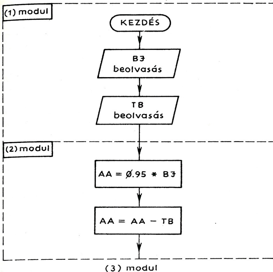
41. ábra. Az (1) és (2) modul folyamata
