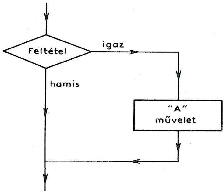
12. ábra. Az IF THEN típusú szerkezet
