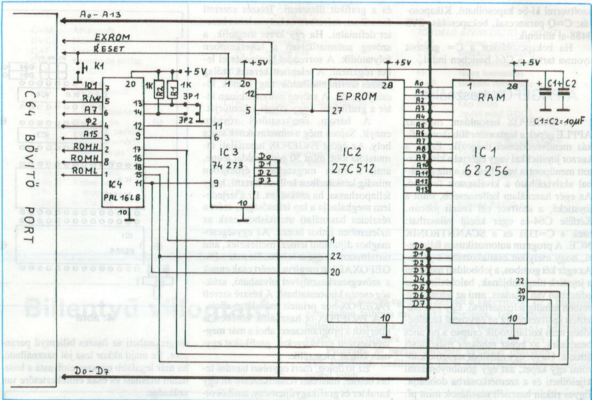
1. ábra A PAGEFOX kapcsolási rajza
