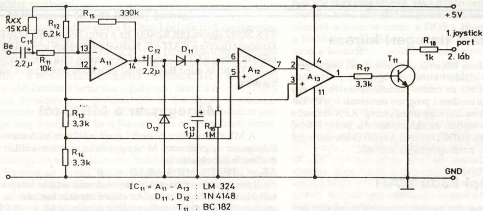
1. ábra A hangkapcsoló kapcsolási rajza
