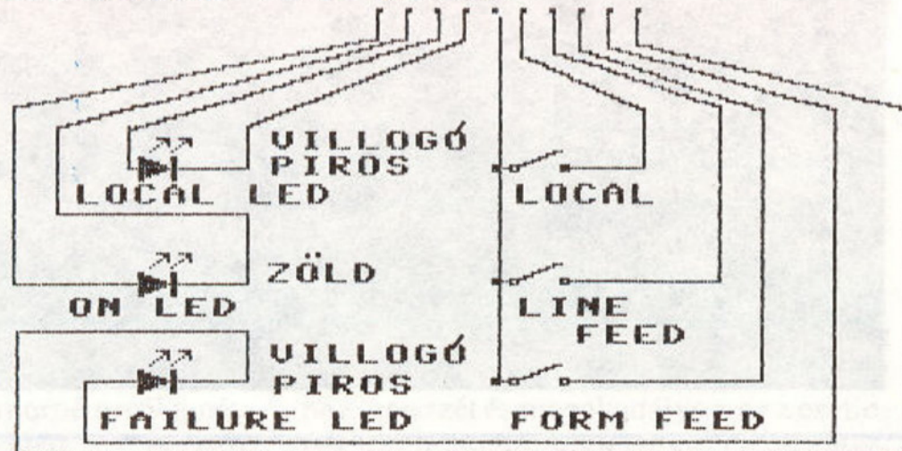
A KIJELZŐK ÉS KAPCSOLÓK BEKÖTÉSE A SZALAGKÁBEL NYÁK FELLŐLI OLDALÁRÓL NEZVE: (COMMODORE MPS 1230)
