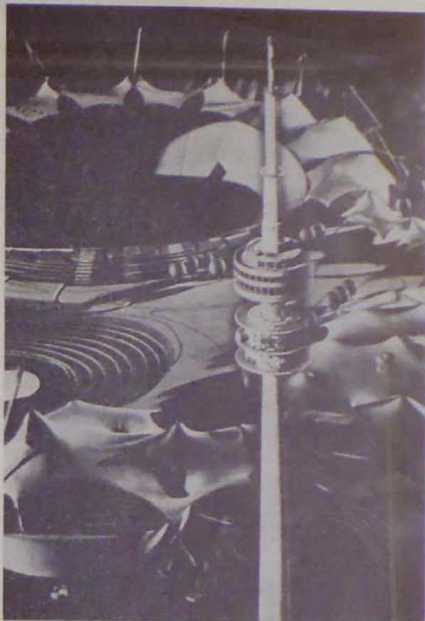
A müncheni Oberwiesefelden álló, majdnem 300 m magas tv-adótorony nemcsak az olimpiai terep jelképe, hanem egyúttal a modern mikrohullámú adástechnika szimbóluma is. A torony hírközlő platformjairól irányított hullámnyalábokat sugároznak Frankfurt, Stuttgart, Nürnberg és Salzburg irányába, valamint a Zugspitzen át Olaszországba. A frankfurti központi elosztóhely adja tovább a tv-programokat az NSZK tv-hálózatának és az Eurovizió-hálózatnak. Frankfurtból mennek az adások a ráis-tíngi Föld-műhold leadóállomáshoz is, amely a Föld fölött „helybenálló” Intelsat típusú mesterséges bolygók közvetítésével az egész világnak továbbítja a programokat.
