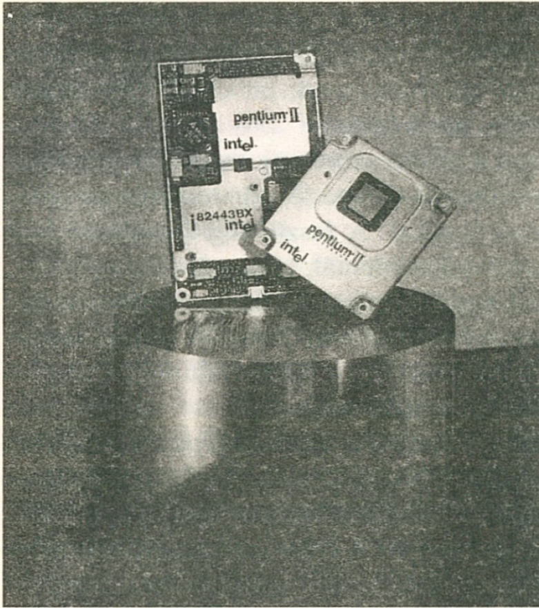
Pentium II mobilmodulban és mini-cartridge-ben – a méretbeli különbség számottevő
