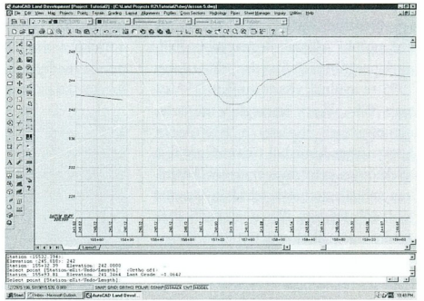
Tervezés hossz-szelvényen
