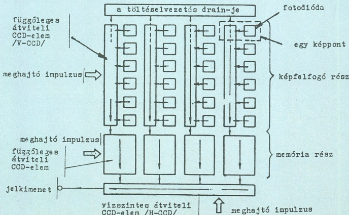
2. ábra. A CCD képzékelő felépítése
